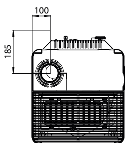
Pohľad zhora
