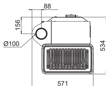
Pohľad zhora
