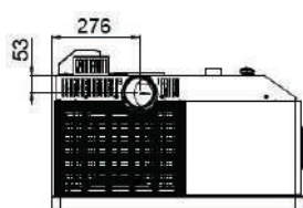
Pohľad zhora
